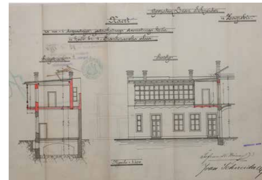
Projekt za dogradnju dvorišnog krila, Šafranek i Wiesner, 1898., DAZ
