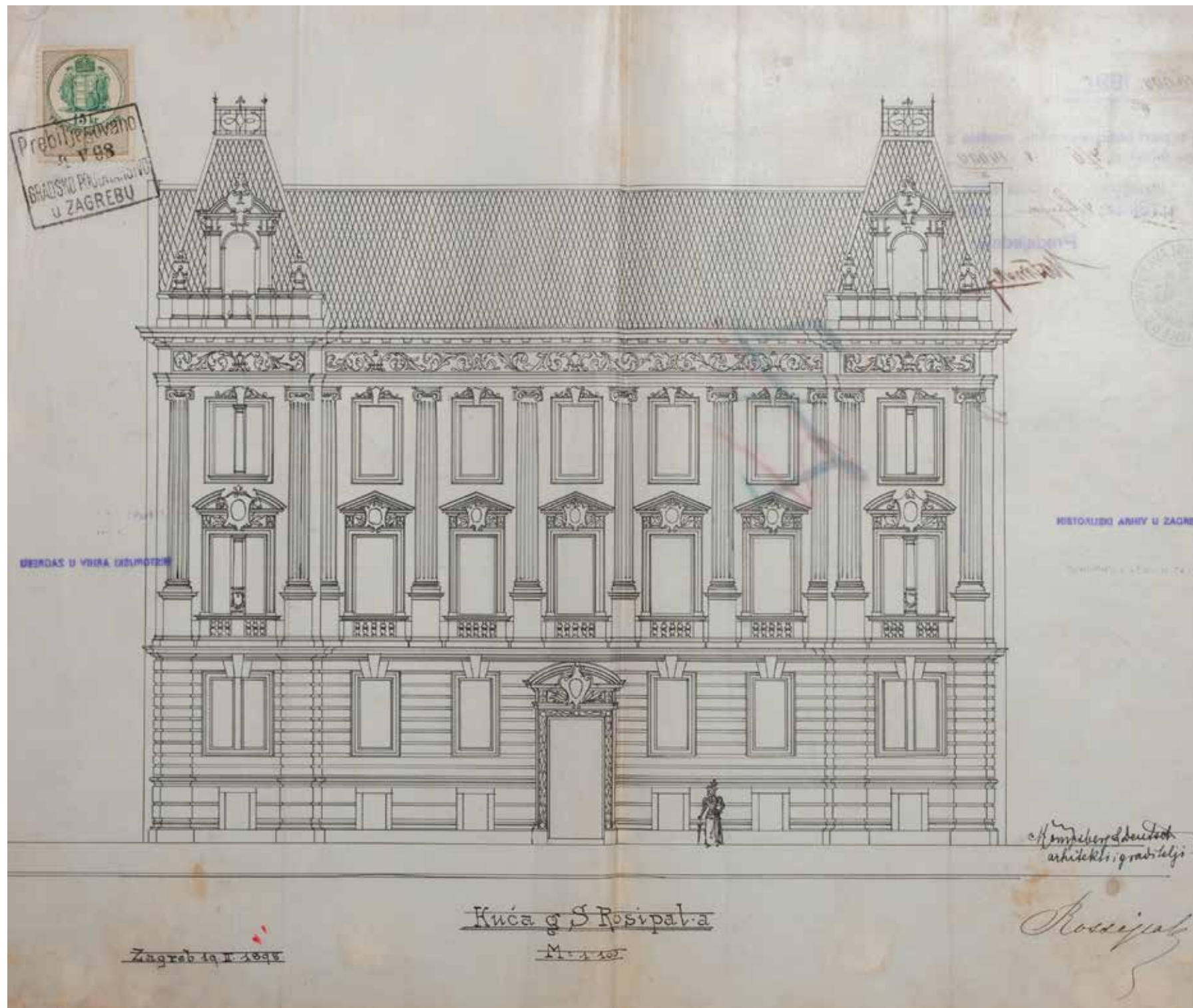
Kuća Rossipal, projekt, Hönigsberg i Deutsch, 1898., pročelje, DAZ
