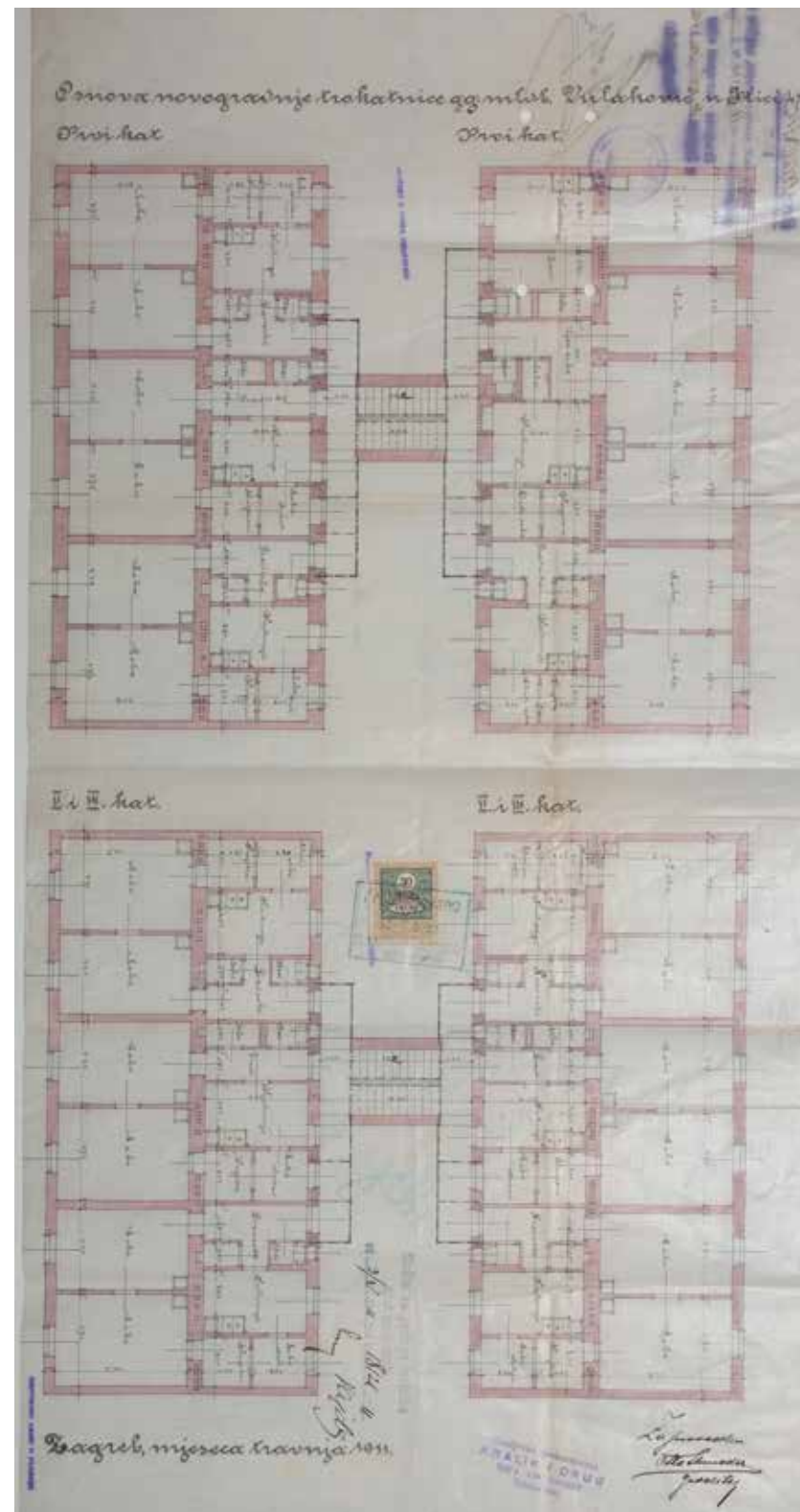
Kuća Vulaković, projekt, Kralik i drug, Amadeo Cernelutti, 1911., tlocrt podruma, prizemlja i katova, DAZ
