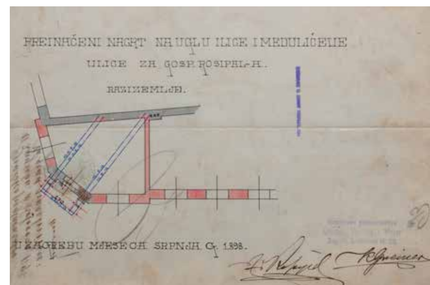
Kuća Rossipal, projekt, Hönigsberg i Deutsch, 1898., situacija i presjek, DAZ
