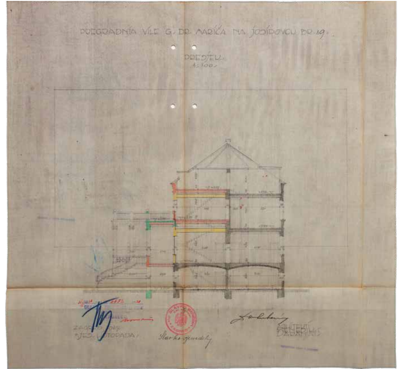
Poprječni presjek, Aladar Baranyai, 1927., DAZG
