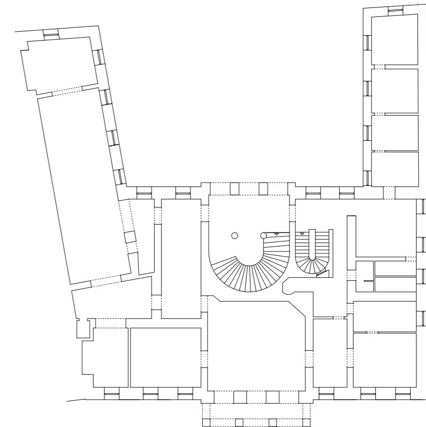
Prizemlje, tlocrt
