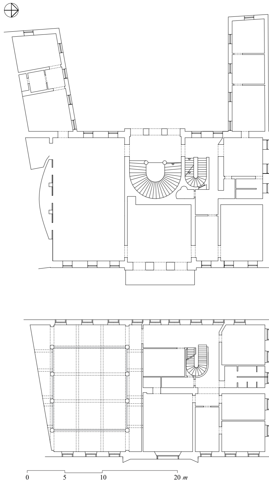
Prvi kat, tlocrt Drugi kat, tlocrt
