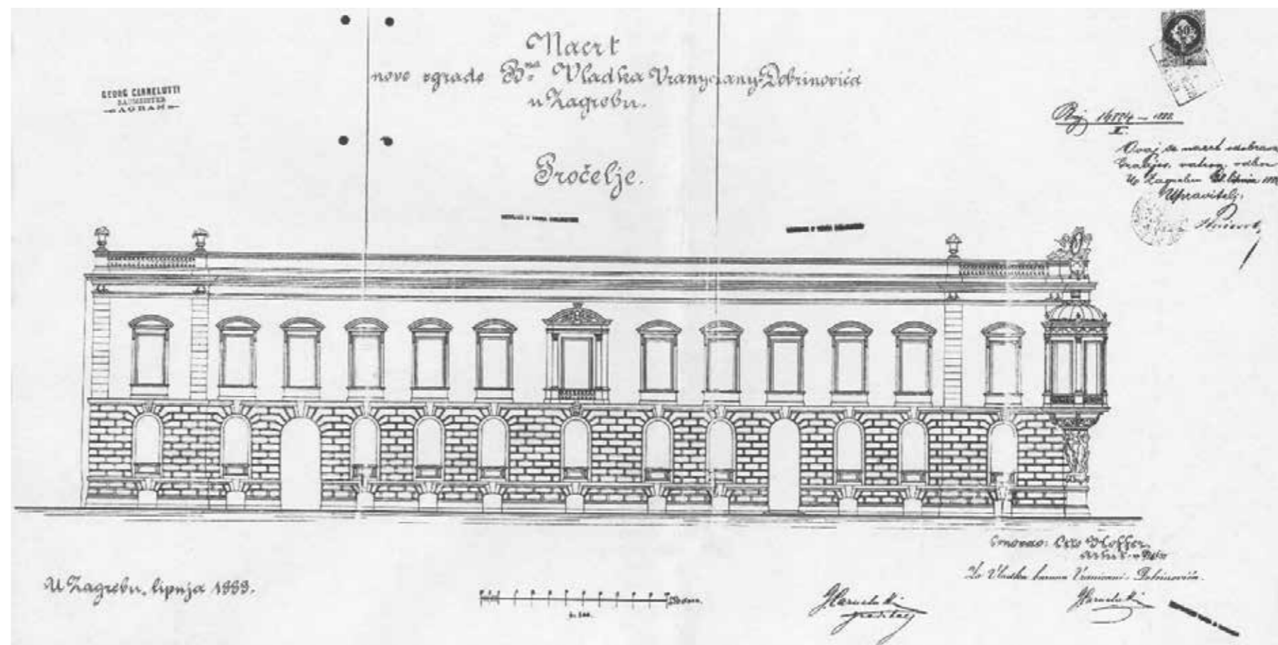
Palača Vladimira Vranyczany-Dobrinovića, Berislavićeva 6–8, projekt pročelja, Otto von Hofer, 1888., DAZG
