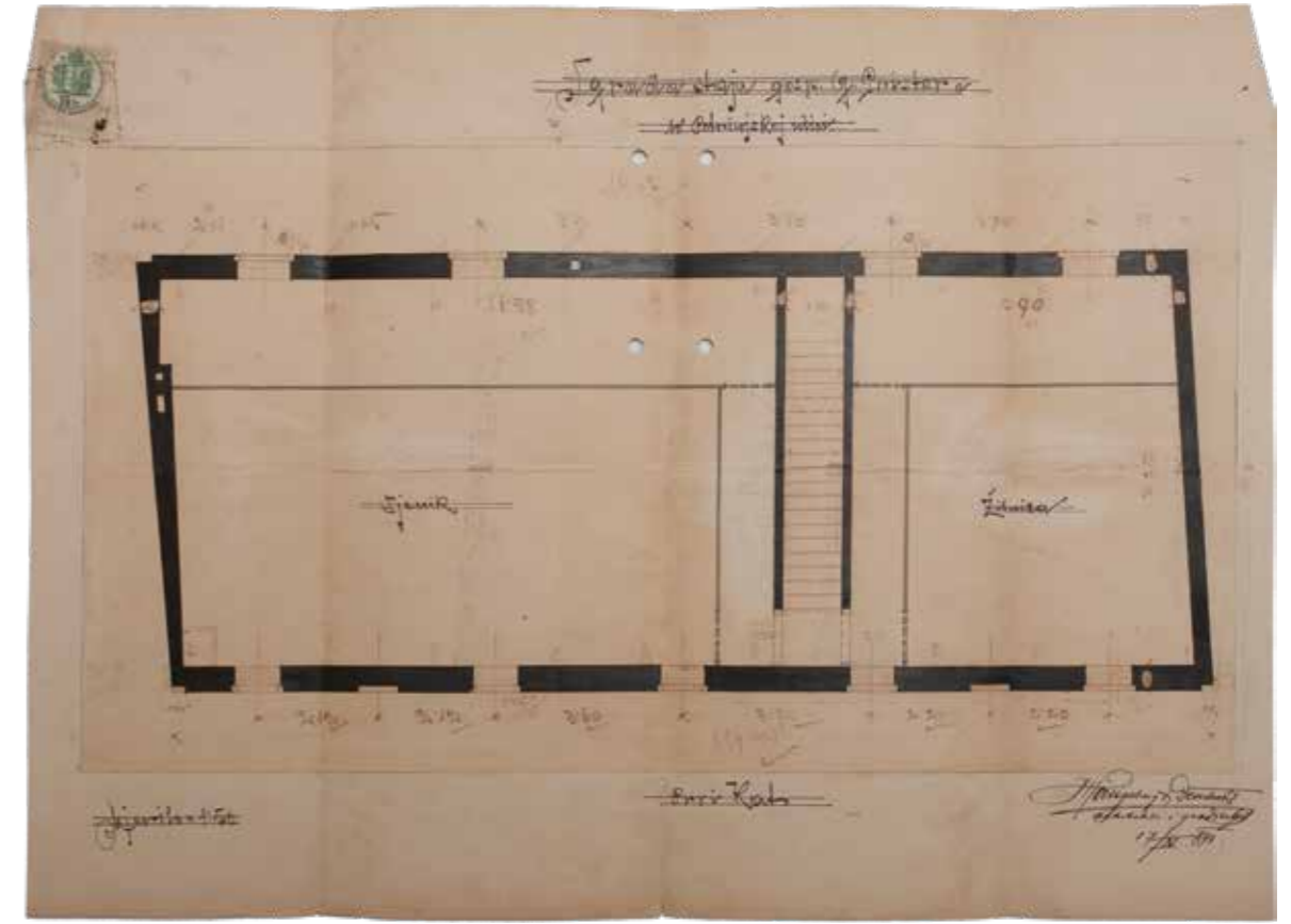
Gospodarska zgrada s konjušnicom, tlocrti podruma, prizemlja i prvog kata, Hönigsberg i Deutch, 17. 4. 1893., DAZG
