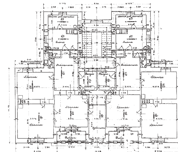
Villa Münz, Akvilejski prilaz 1, tlocrt prizemlja.
