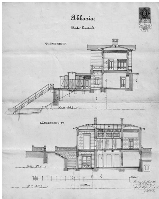
Opatija, Nacrtn Kupališnog zavoda s prvom fazom kupališta Angiolina (bočni i uzdužni presjek), HR-DARI-0029, Glavarstvo općine Volosko – Opatija, Građevinski arhiv, Opatija 33, potpisnik nacrtFranz Wilhelm.
