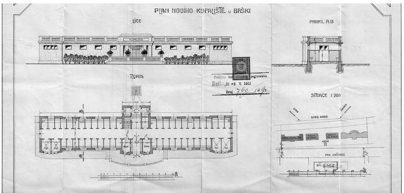
Baška, Nacrtnovog kupališta u Baški, HR-DARI-0024, Glavarstvo općine Baška, spis br. 760/1911, 1911. godina
