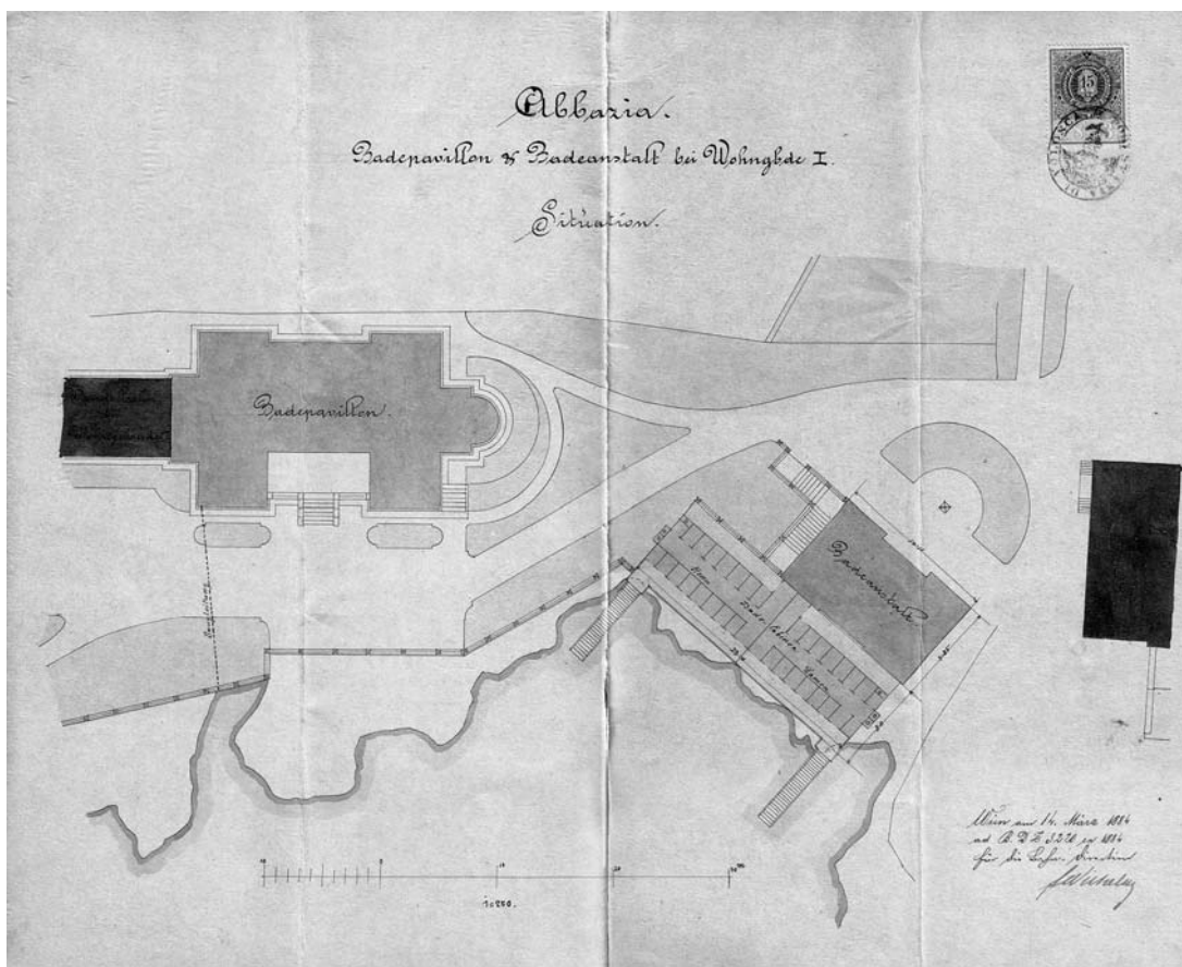
Opatija, Nacrta situacije: Kupališni paviljon hotela Kvarner, Kupališni zavod s kupalištem Angiolina, HR-DARI-0029, Glavarstvo općine Volosko – Opatija, Građevinski arhiv, Opatija 33, potpisnik nacarta Franz Wilhelm (dvojno stepenište za ulazak u more s kupališta nije realizirano kako je predviđeno projektom, op.a.)
