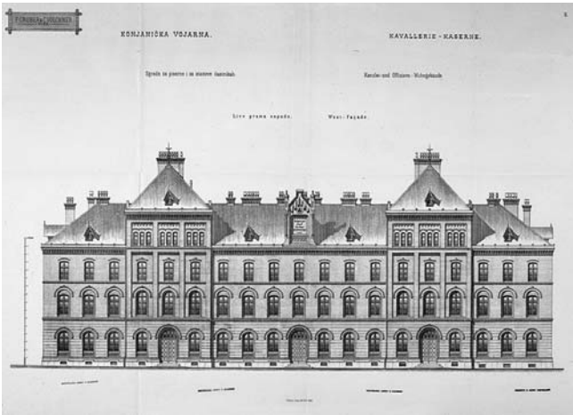
7. F. Gruber i F. Völckner, Nacrt zapadnog pročelja glavne zgrade konjaničke vojarnice (na Draškovićevoj ulici), 1881/1882. (atr.)
