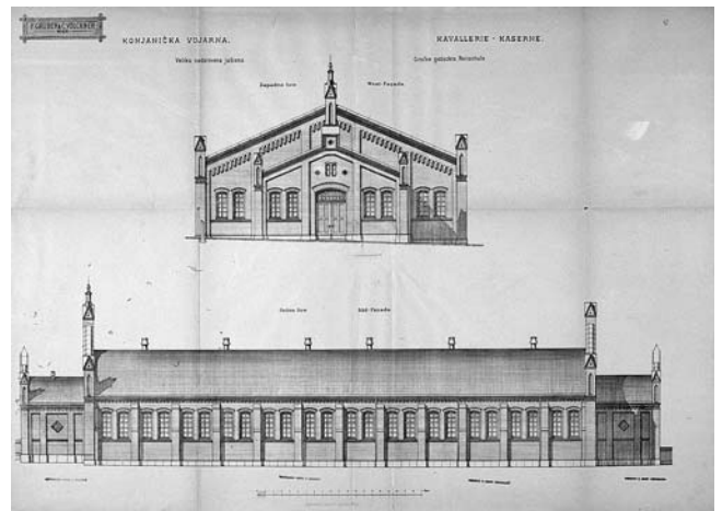
8. F. Gruber i F. Völckner, Nacrt zapadnog i južnog pročelja velike natkrivene jašione konjaničke vojarnice, 1881./1882. (atr.)
