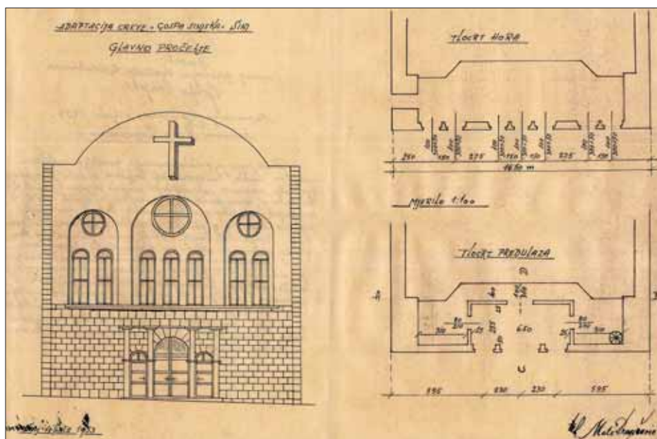
Projekt za novo crkveno pročelje, Mate Dragičević, 1953. (AFSS, Fond nacrtu)
