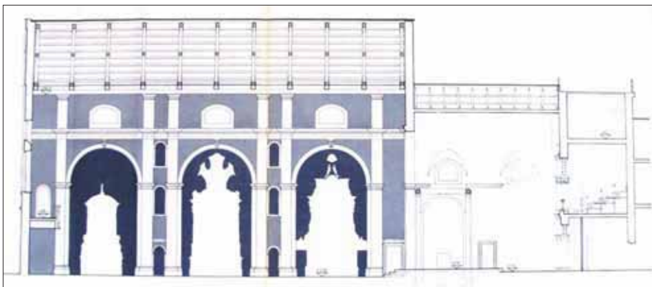
Uzdužni presjek unutrašnjosti crkve, Bernardo Bernardi, 1974. (AFSS, Fond nacrt)
