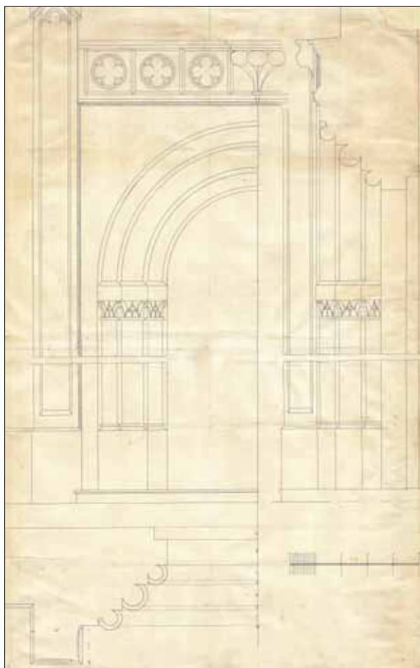
Detalji portala novog crkvenog pročelja, Karlo Beckmann, 1862. (AFSS, Fond nacrt)
