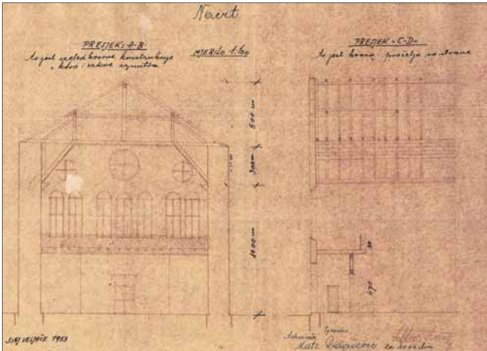
Projekt za novo crkveno pročelje – poprečni i uzdužni presjek, Mate Dragičević, 1953. (AFSS, Fond nacrtu)
