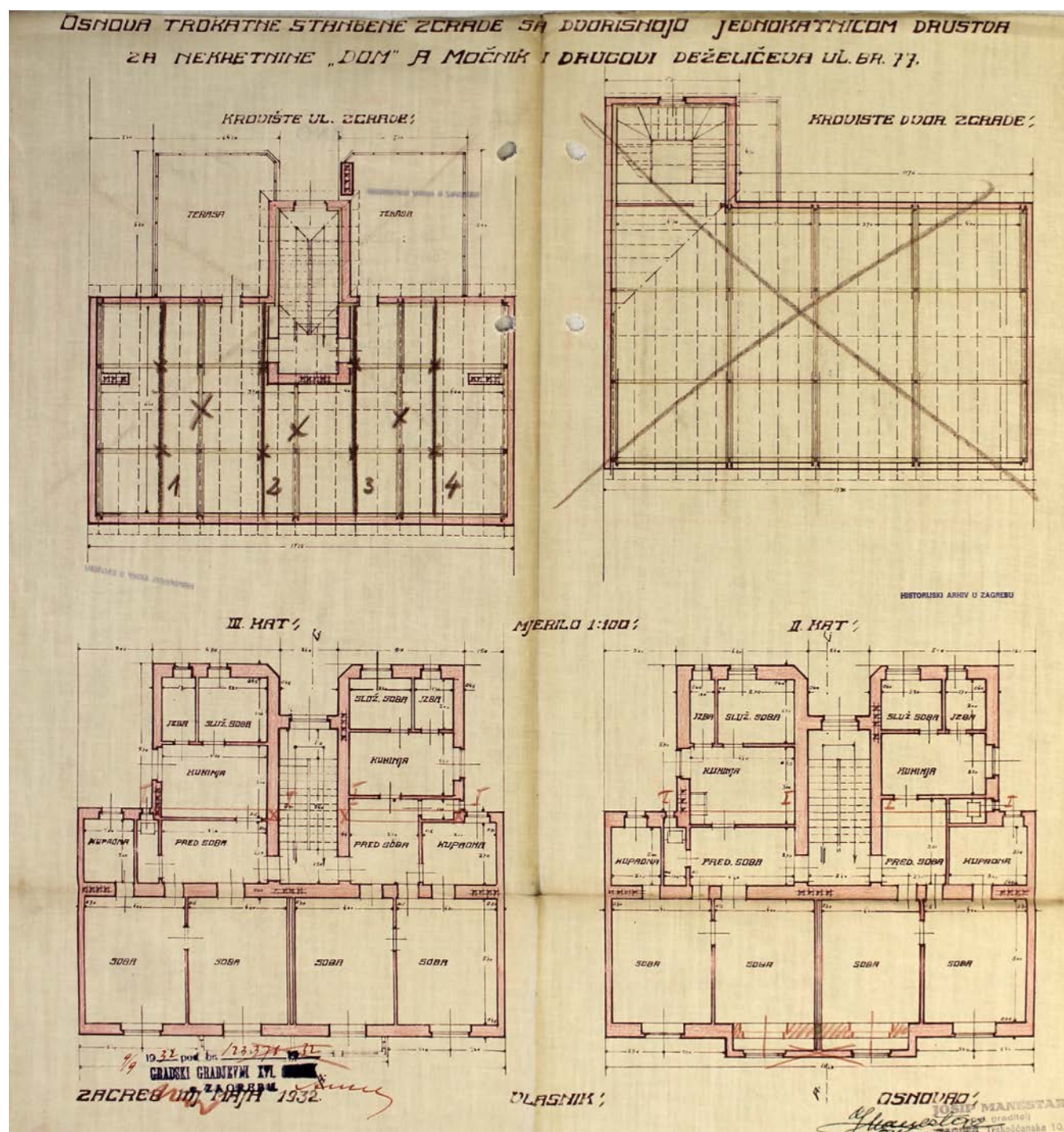
Sl. 47. Projekt za stambenu troklatnicu i dvorišnu jednokatnicu s dvoranom, kroviste i katovi, Josip Manestar, svibanj 1932. (DAZG)
