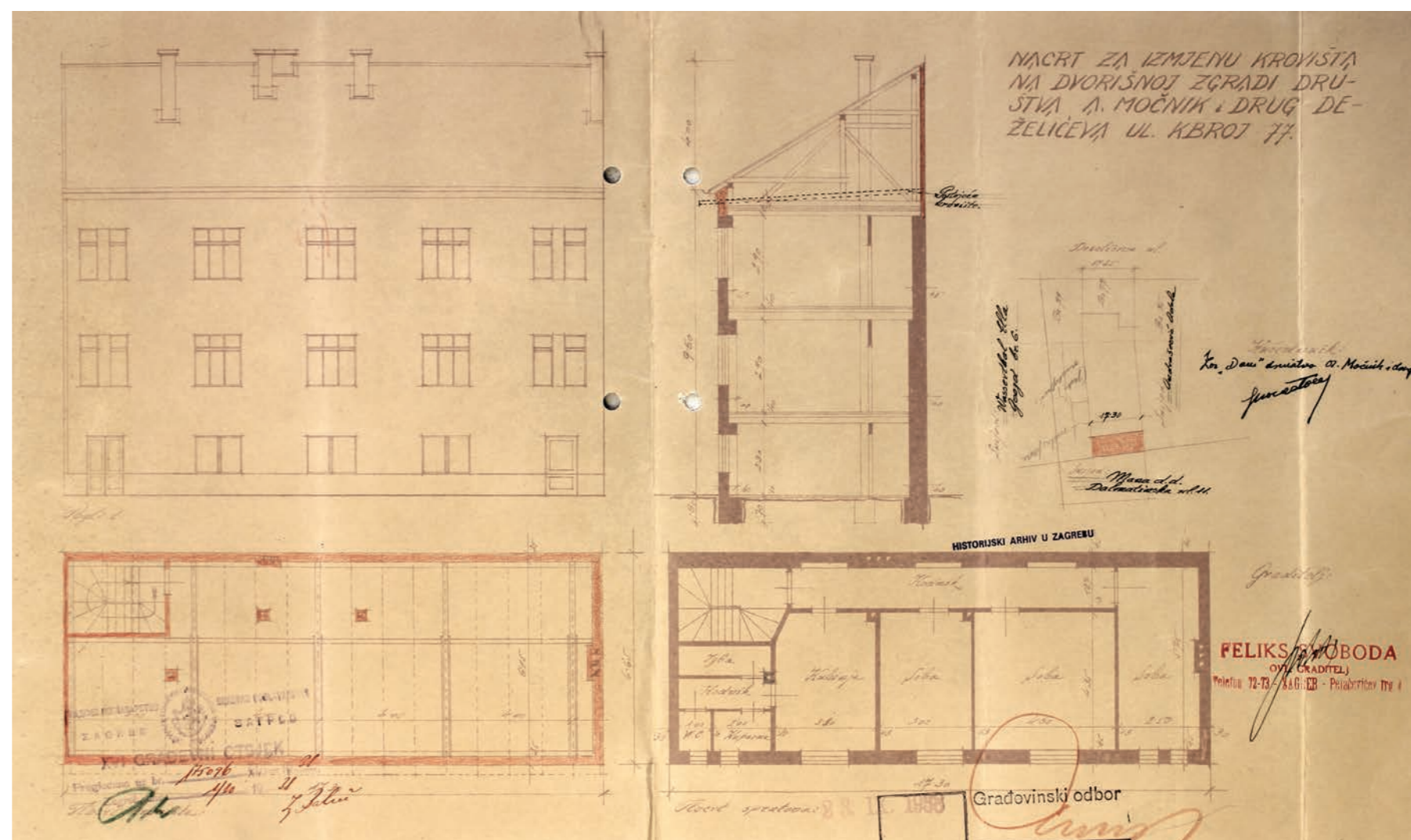
Sl. 60. Projekt za preoblikovanje krovista dvorišne dvokatnice, glavno pročelje, presjek, tlocrt krovista i karakterističnog kata te situacija, Feliks Svoboda, rujanj 1938. (DAZG)
