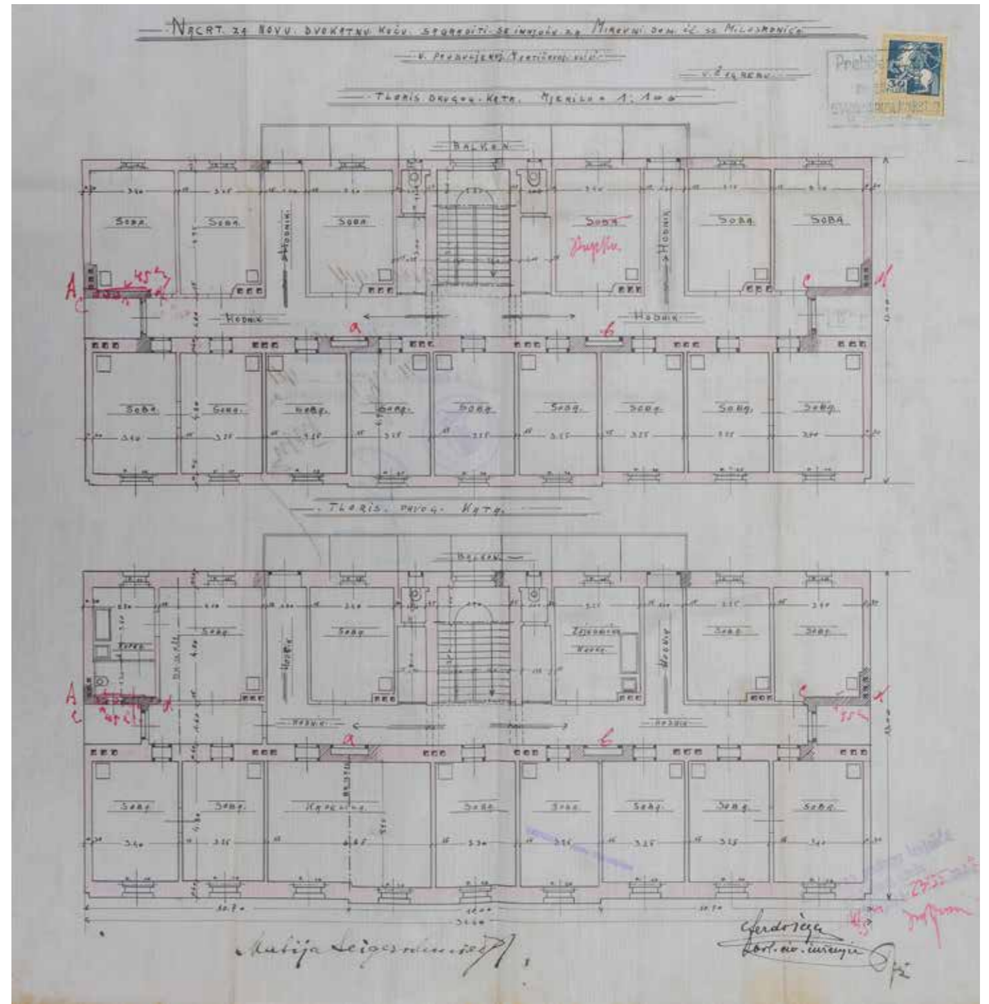
Mirovni dom sestara milosrdnica, tlocrt podruma, prizemlja i katova, projekt, ing. Ferdo Šega, 1914., Državni arhiv u Zagrebu
