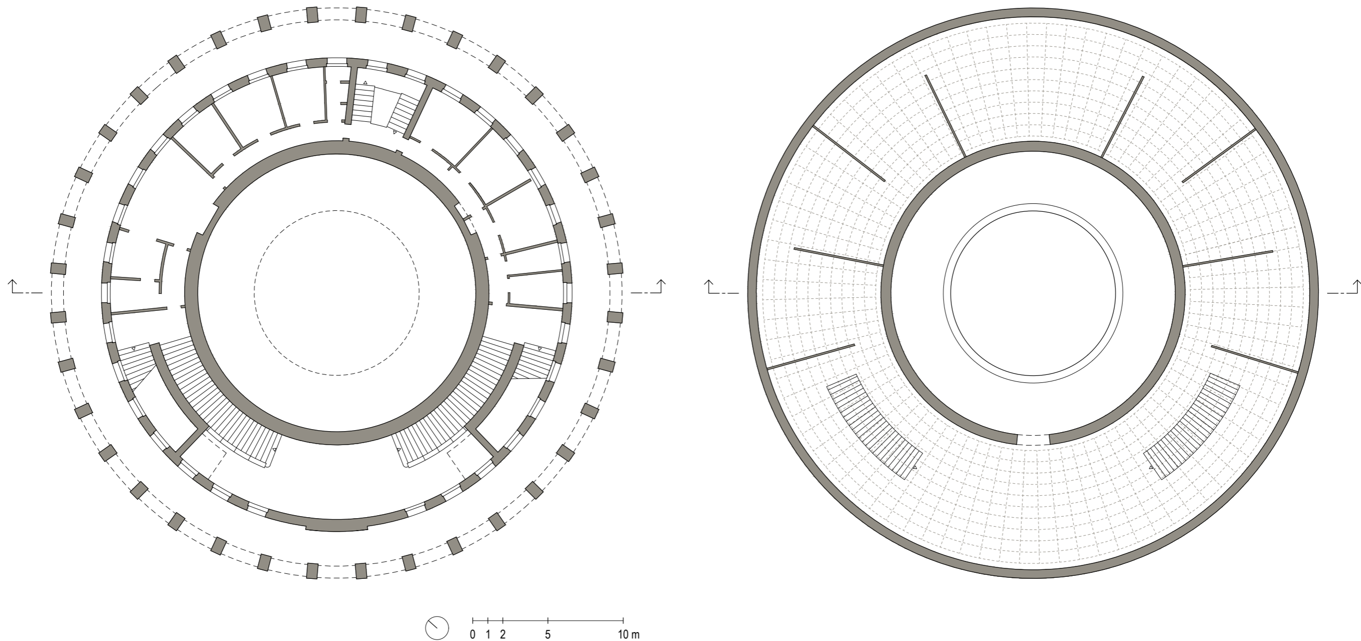
Tlocrt mezanina
