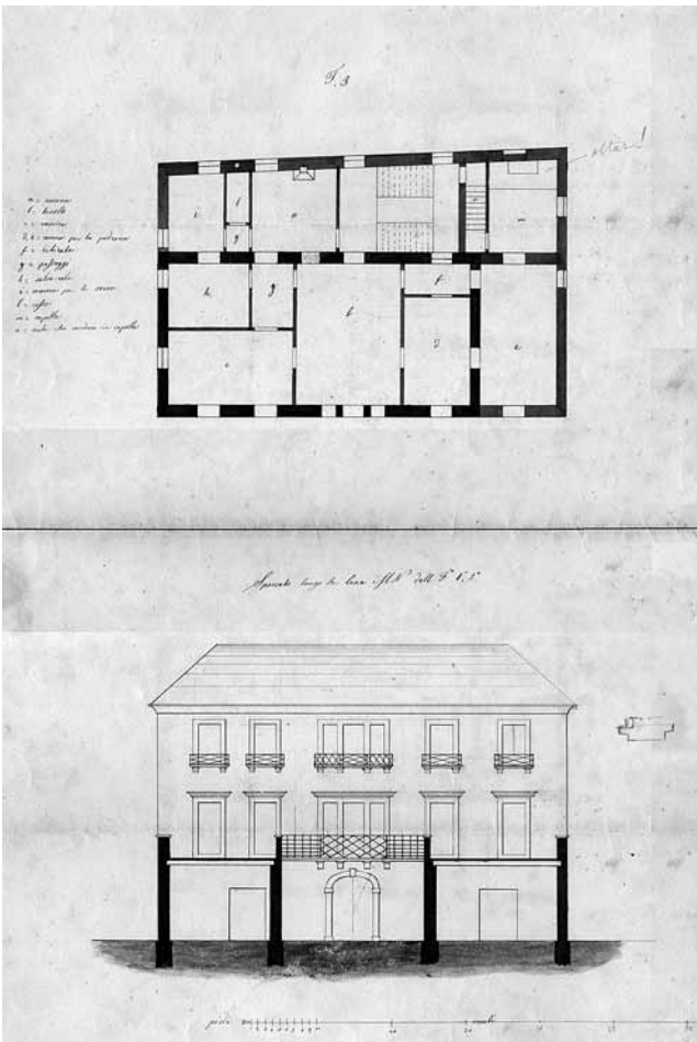
8. Projekt adaptacije Josipa Slade, tlocrt 2. kata i presjek kroz gospodarske prizemnice s pogledom na glavno pročelje kuće (DAS, FSS)
