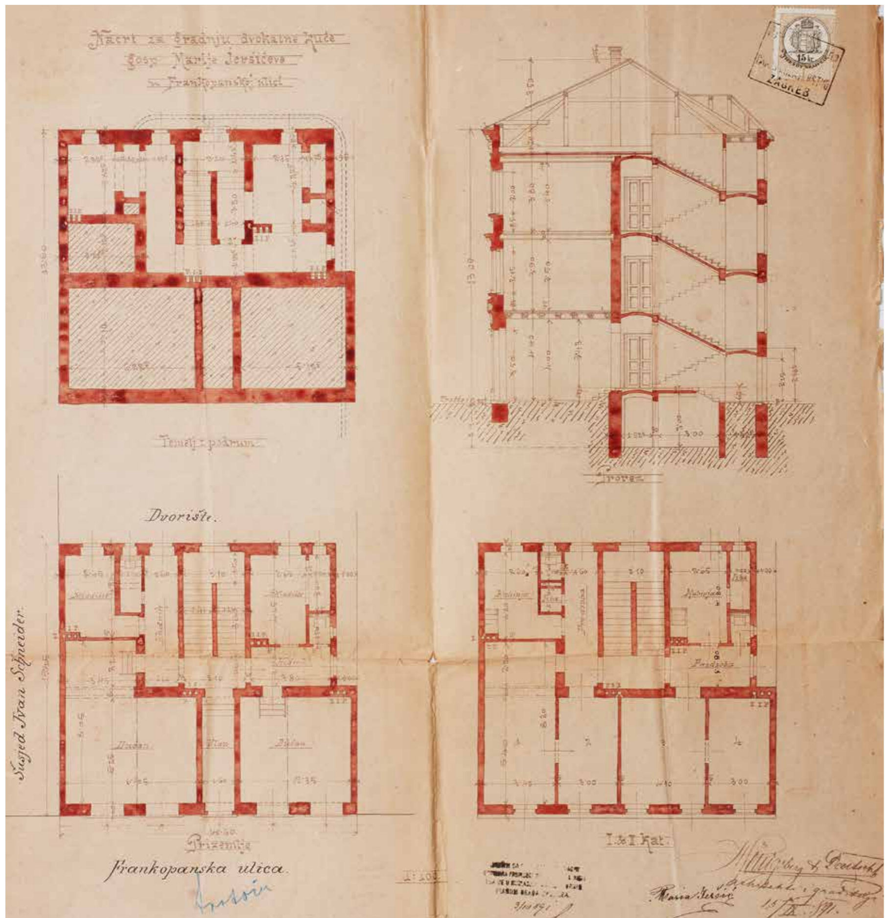
Kuća Jeršić, projekt, Hönigsberg i Deutsch, 1891., tloct podruma, prizemlja i katova, presjek kroz stubište, DAZ
