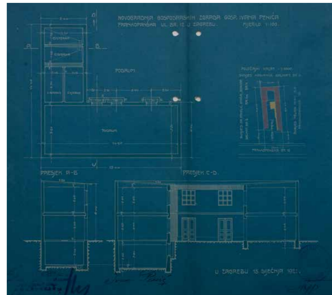
Projekt dogradnje dvorišnih zgrada, Mauricij Stapp, 1921., DAZ
