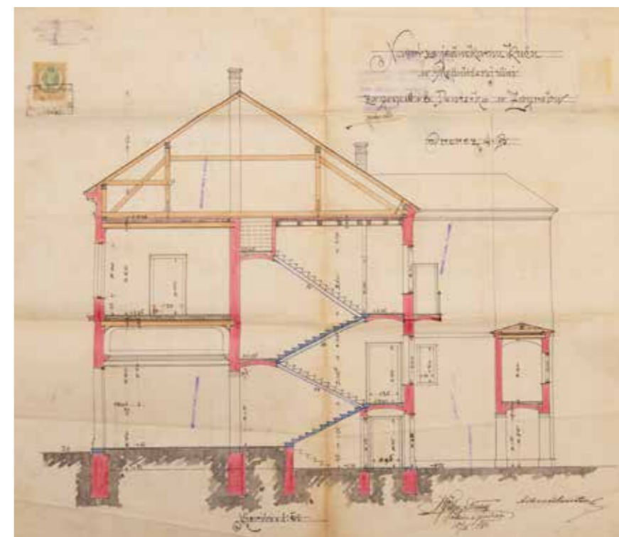
Kuća Deutsch, projekt, Hönigsberg i Deutsch, 1893. presjek, DAZ
