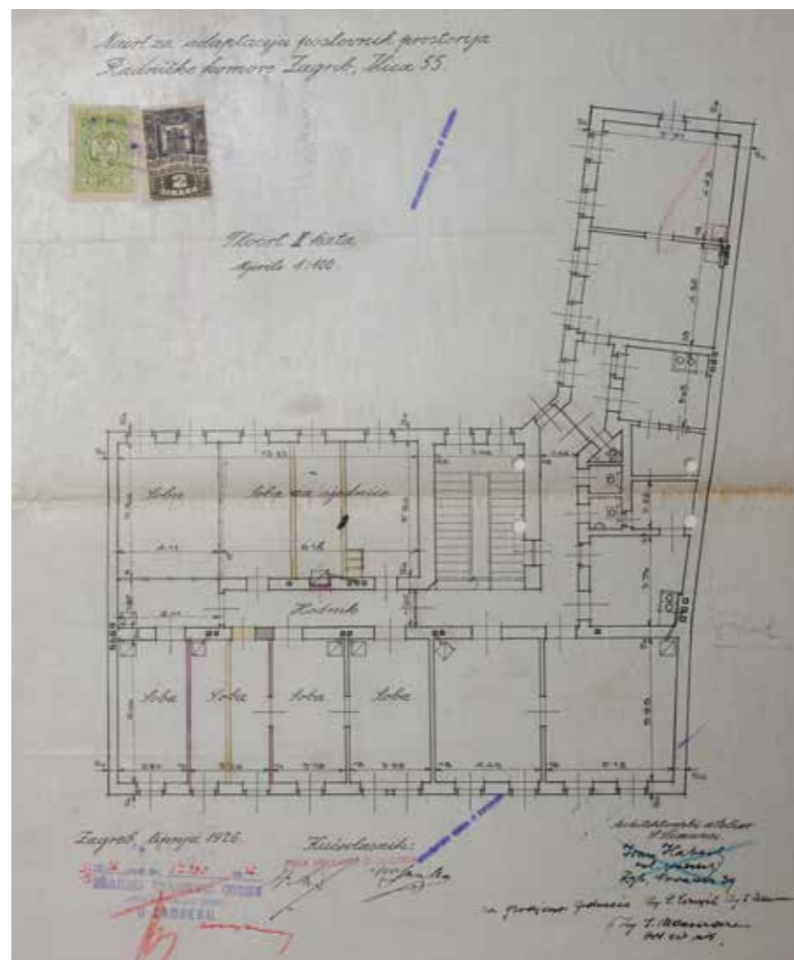
Kuća Rath, projekt prenamjene stambenih prostorija u poslovne prostorije Radničke komore, Svetimir Šimunec, 1926., tlocrt prvog i drugog kata, presjek, DAZ
