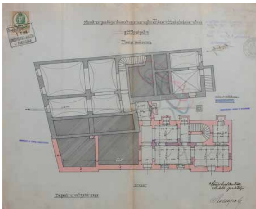
Kuća Rossipal, projekt, Hönlingsberg i Deutsch, 1898., tlocrt prizemlja, podruma i katova, DAZ
