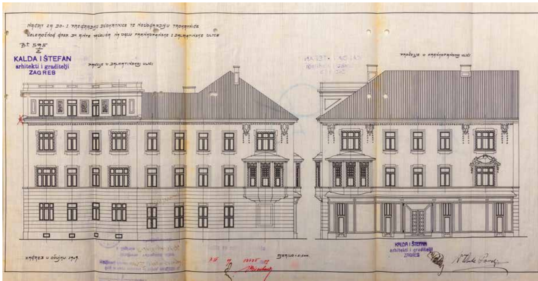
Kuća Pavelić, projekt, Lav Kalda 1909., južno i istočno pročelje, DAZ
