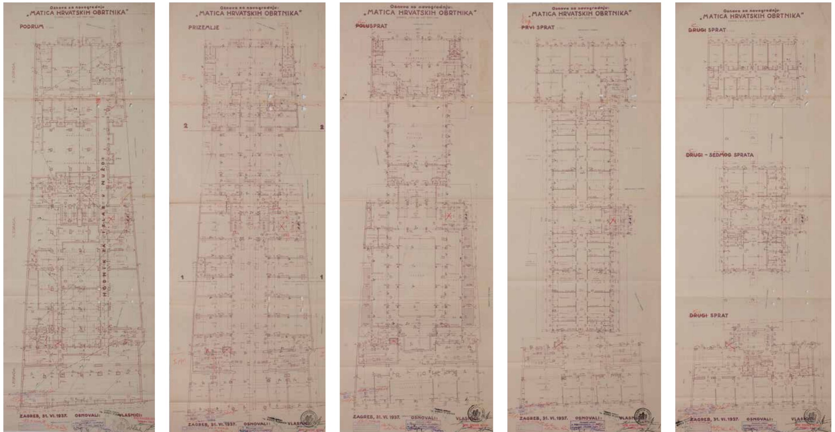
Matica hrvatskih obrtnika, projekt, Aleksandar Freudreich i Zvonimir Požgaj, 1937., tlocrt podruma, prizemlja, polukata i katova, DAZ
