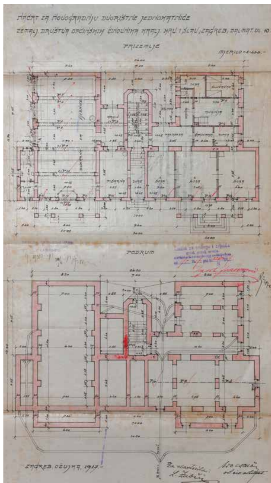
Zgrada zemaljskog društva općinskih činovnika, projekt, Edo Schön, 1917., tlocrt podruma i prizemlja, presjeci, DAZ
