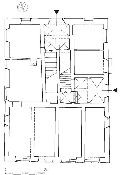
Prva općinska kuća na Placi, tlocrt prizemlja i pročelje, arhitektonska snimka: Ivan Tenšek, Ivana Valjato-Vrus
