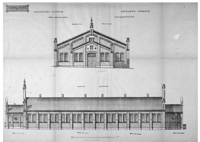
8. F. Gruber i F. Völckner, Nacrt zapadnog i južnog pročelja velike natkrivene jašione konjaničke vojarnu, 1881/1882. (atr.)
