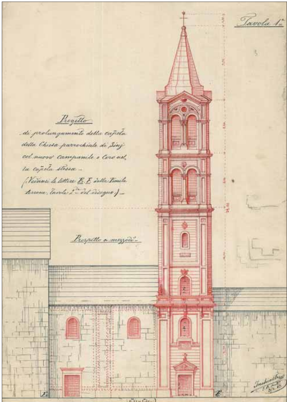
Prijedlog za izgradnju novog zvonika G. B. A. Inchiostru, veljača 1887. (AFSS, Fond nacrtu)
