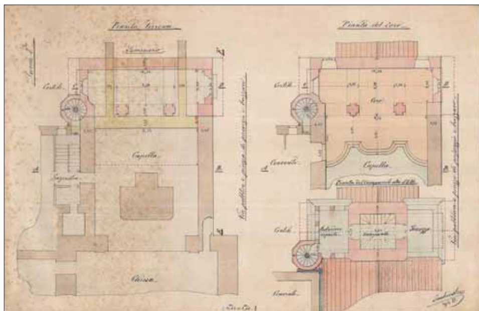
Projekt novog redovničkog kora i zvonika, G. B. A. Inchiostri, siječanj 1887. (AFSS, Fond nacarta)
