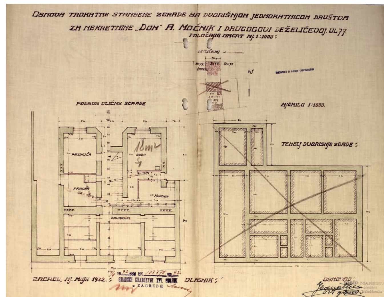
Sl. 48. Projekt za stambenu trokutnicu i dvorišnu jednokatnicu s dvoranom, podrum glavne ulične i temelji dvorišne zgrade, Josip Manestar, svibanj 1932. (DAZG)
