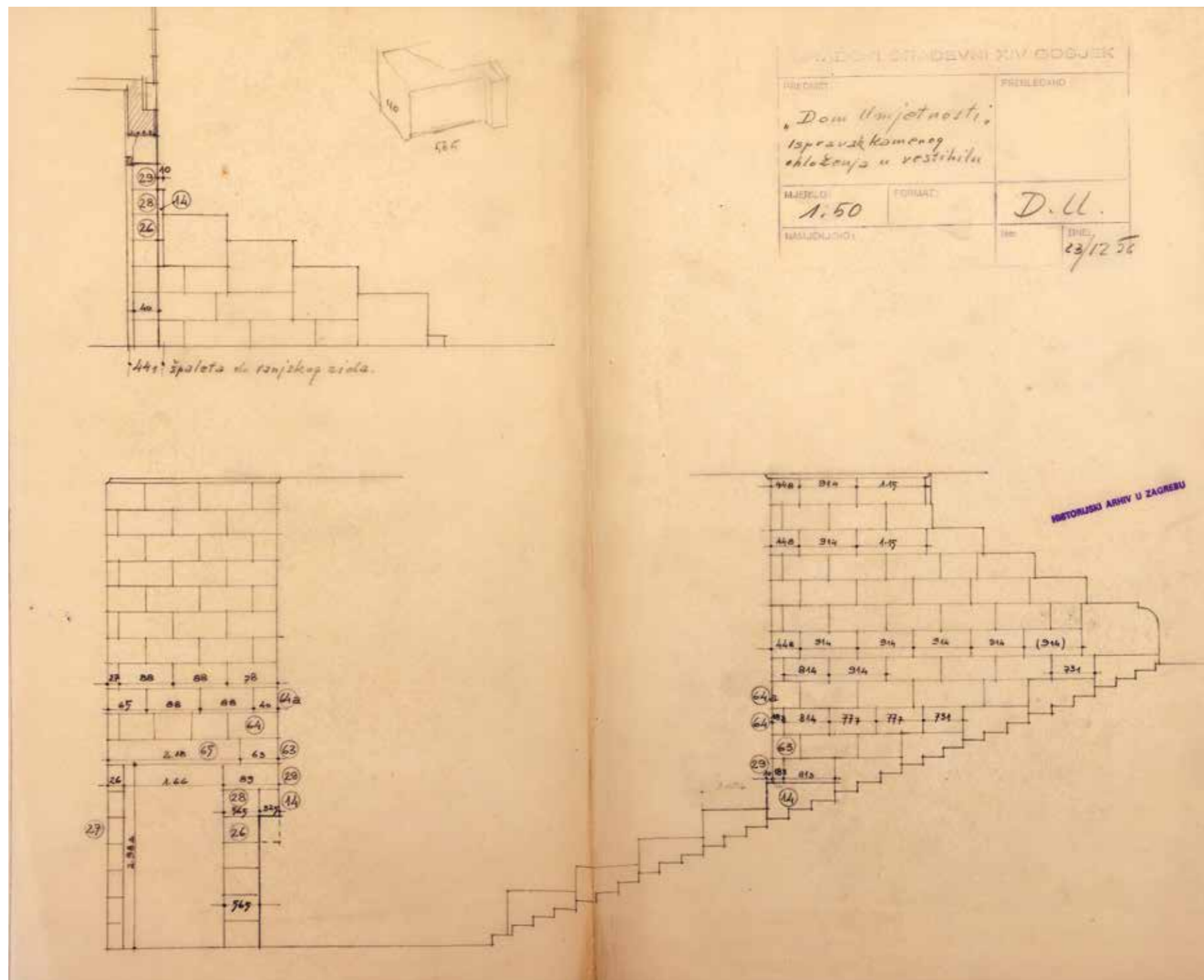
Nacrt oblaganja kamenih ploča u vestibulu, DAZG
