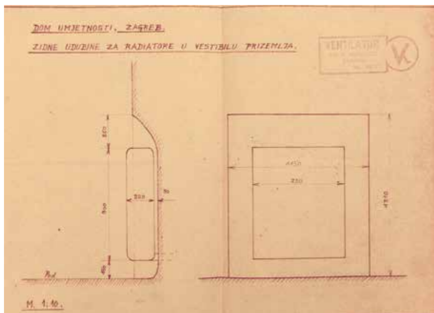
Nacrt zidnih udubina za radijatore u vestibulu prizemlja, DAZG
