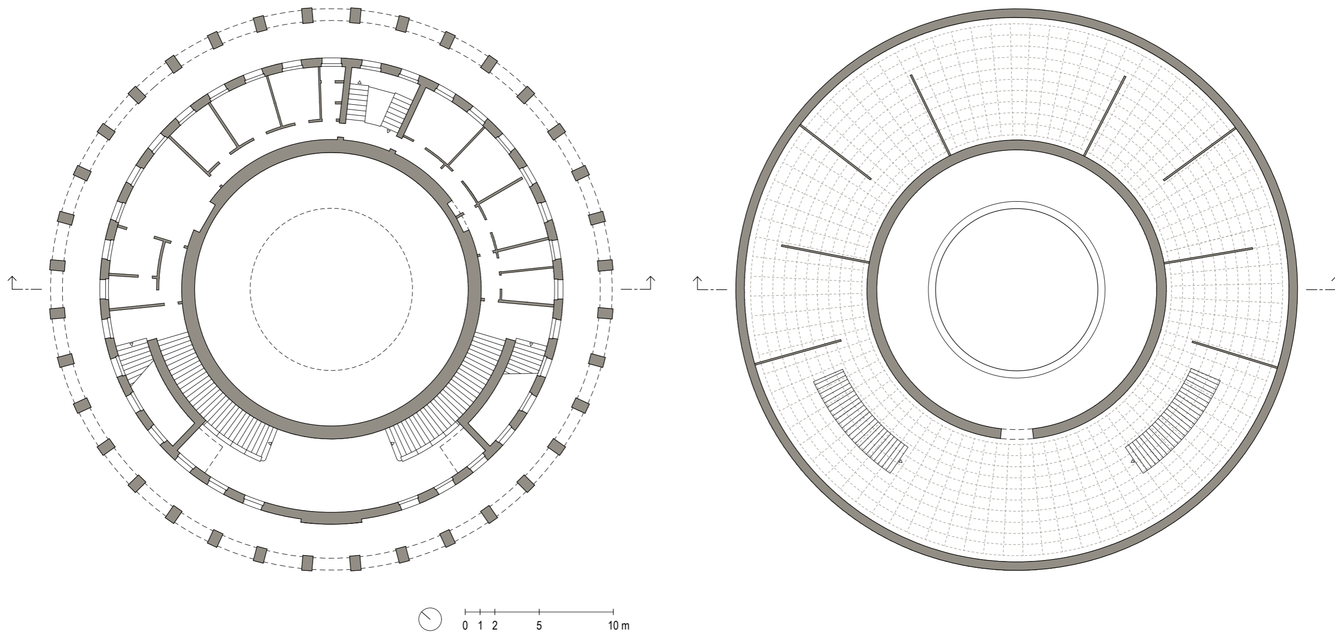
Tlocrt mezanina
