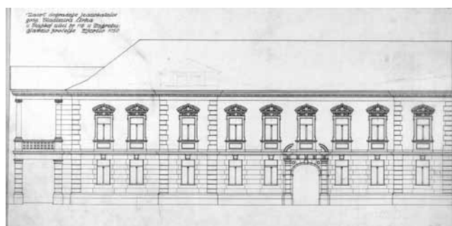
8. Ignjat Fischer, rezidencija i poslovница Vladimira Arka, Vlaška 116, Zagreb, 1918., nacrt glavnoga pročelja (Hrvatski državni arhiv, Zagreb, Zbirka nacrti)
