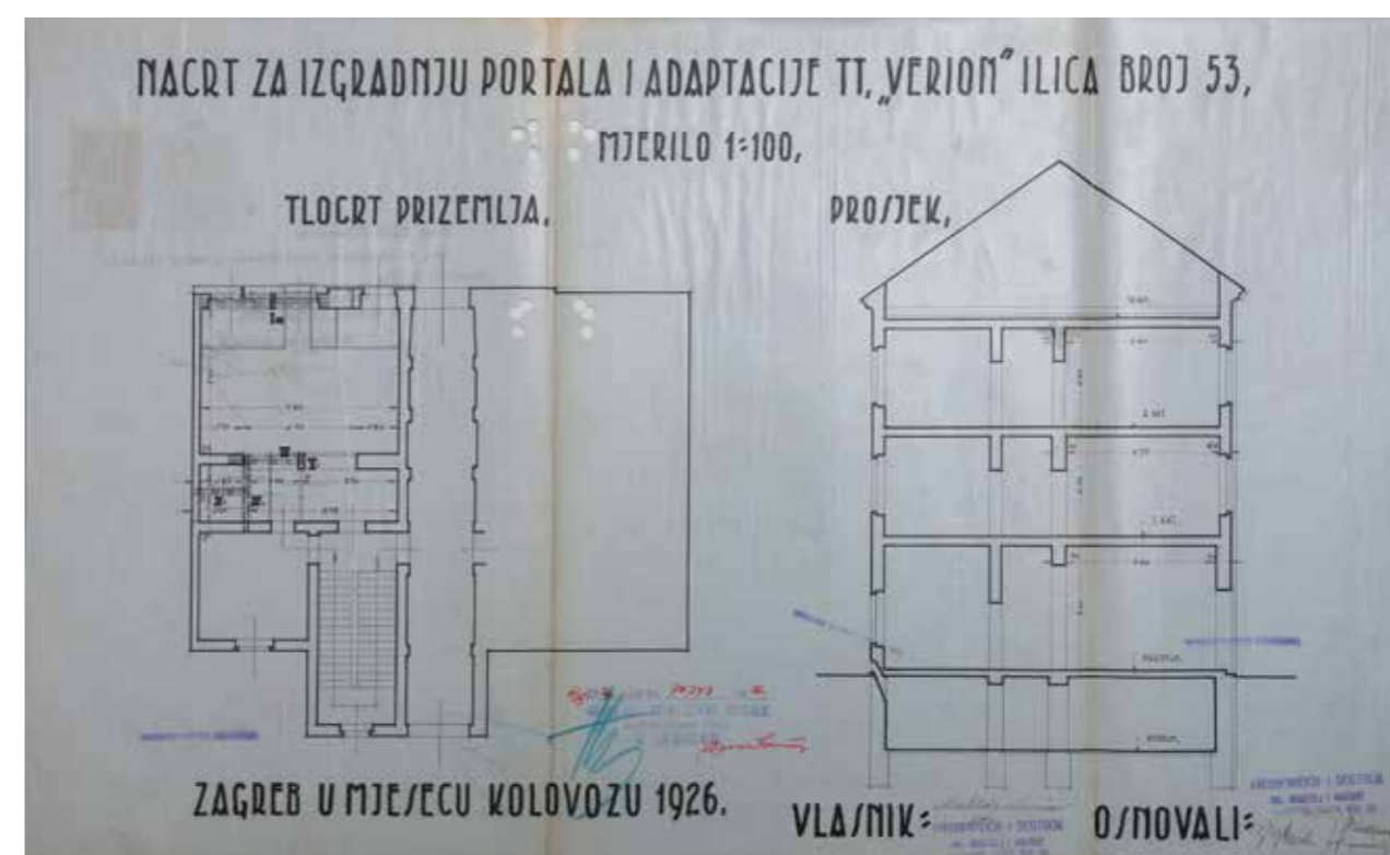
Projekt pregradnje prizemlja (br. 53), 1926., DAZ
