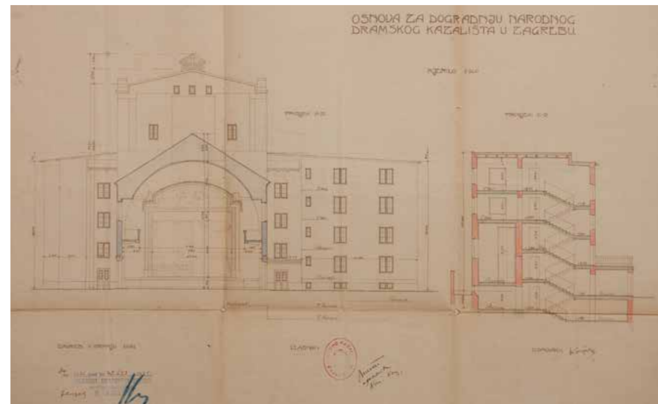
Malo kazalište u Frankopanskoj, Josip Dryak, 1921., presjeci, DAZ
