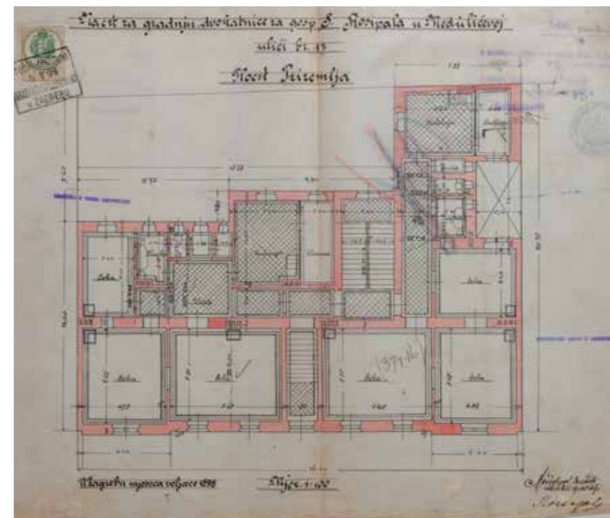
Kuća Rossipal, projekt, Hönigsberg i Deutsch, 1898. (neizvedena varijanta), situacija i tlocrt prizemlja, DAZ
