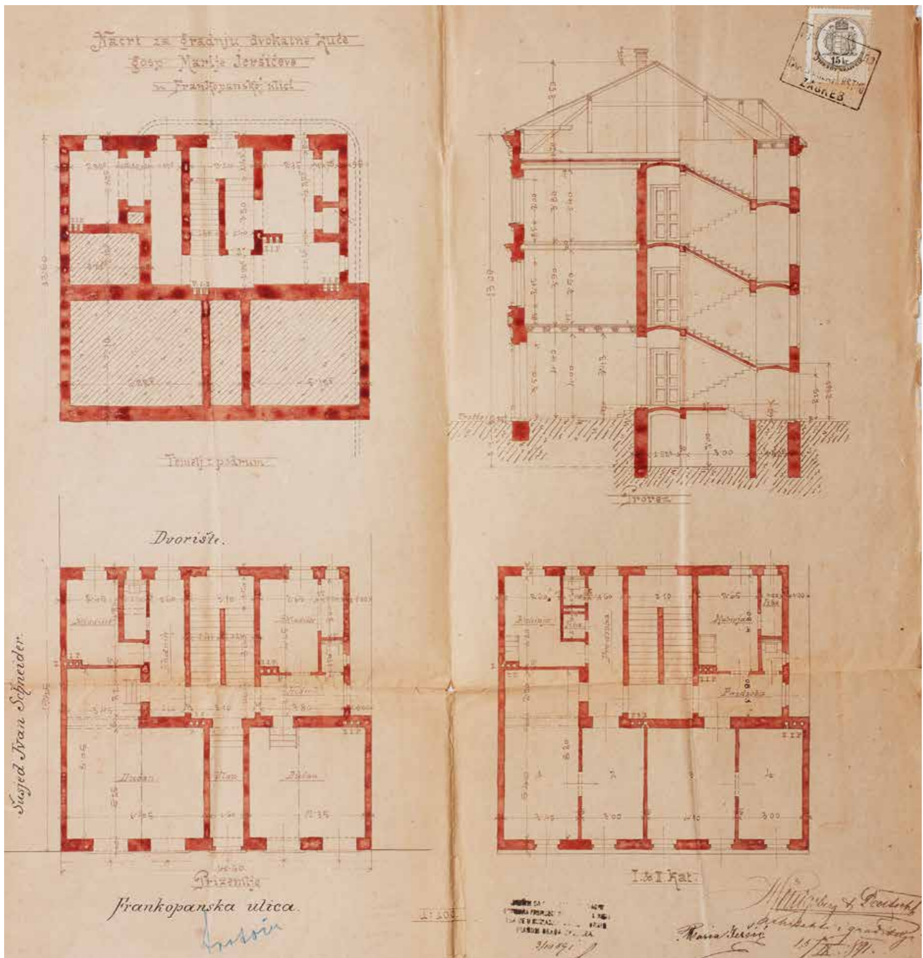
Kuća Jeršić, projekt, Hönigsberg i Deutsch, 1891., tlocrt podruma, prizemlja i katova, presjek kroz stubište, DAZ
