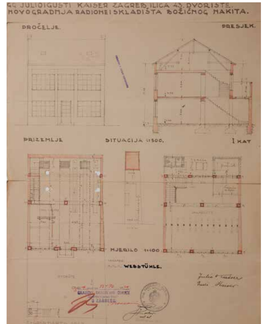
Radionica i skladište božićnog nakita, projekt, Moses Lorber, 1929., pročelje, presjek, tlocrt prizemlja i kata, DAZ
