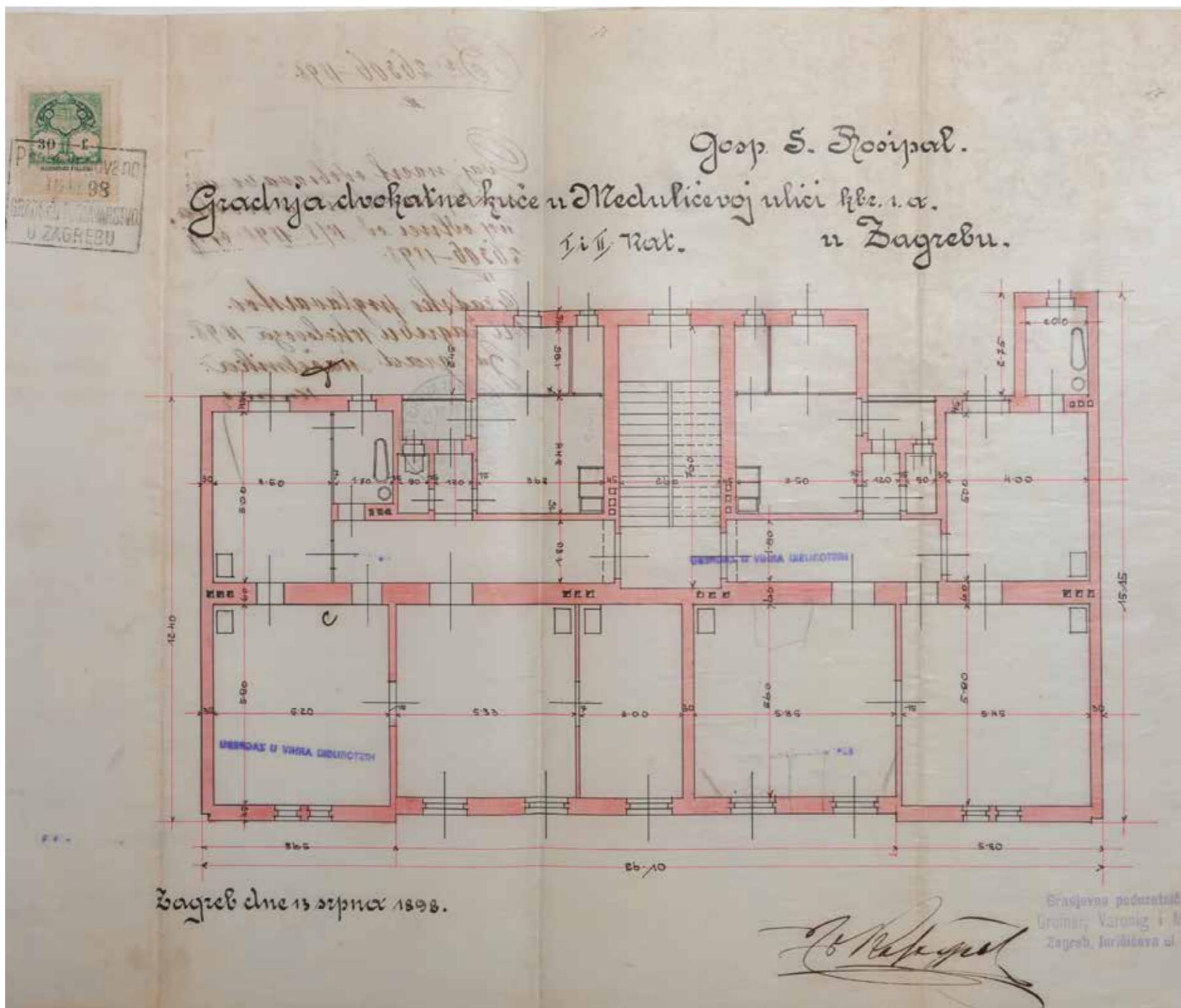
Kuća Rossipal, projekt Hönlberg i Deutsch, 1898. (izvedena varijanta), tlocrt prizemlja i katova, DAZ
