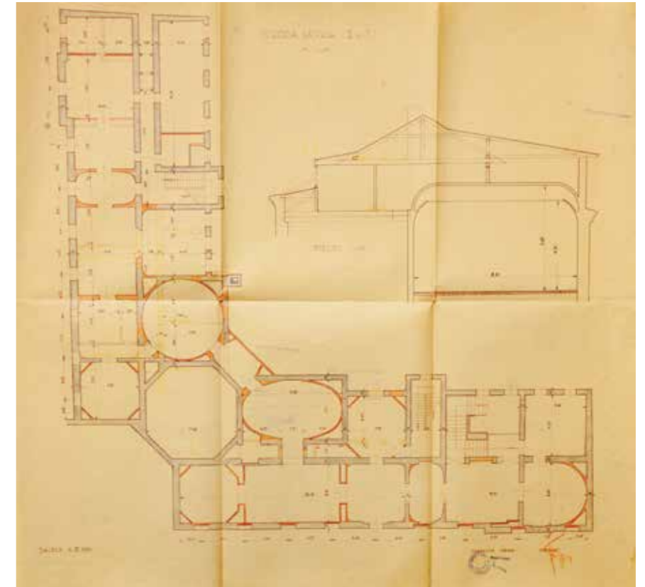
Nacrt pregradnje drugog kata sjevernog krila za Modernu galeriju, Ivo Župan, 1950., DAZG
