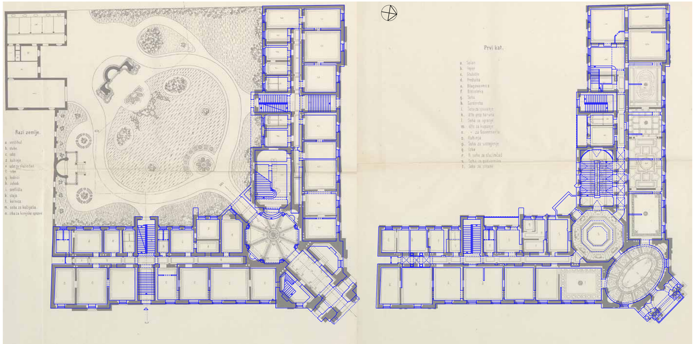
TLOCRT PRIZEMLJA
