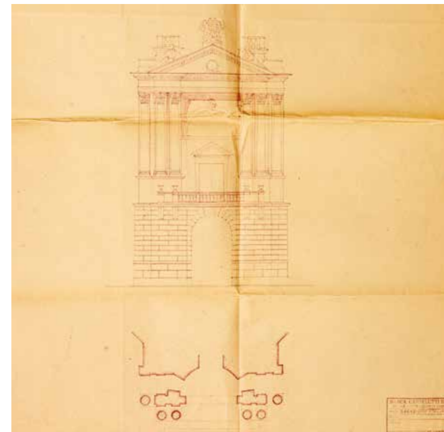
Nacrt rizalita palače za Legazione Italiana , braća Carnelutti, 1941., DAZG
