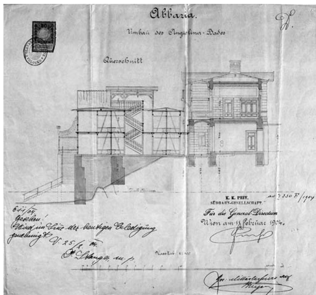
Opatija, Nacrt dogradnje kata na kupalištu Angiolina, HR-DARI-0029, Glavarstvo općine Volosko – Opatija, Građevinski arhiv, Opatija 33, potpisnik nacrtu Alois Breyer.
