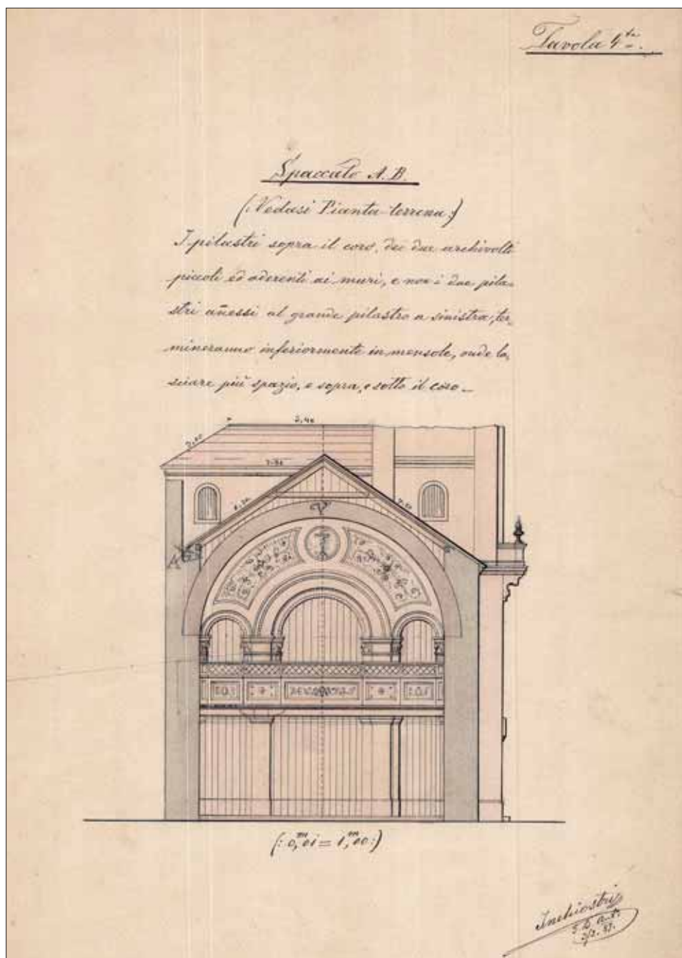
Prijedlog novoga redovničkog kora, G. B. A. Inchiestri, veljača 1887. (AFSS, Fond nacrtu)
