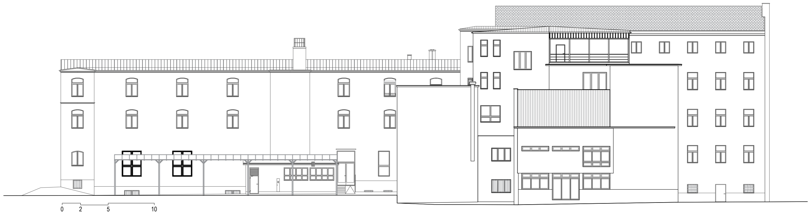
Južno pročelje
