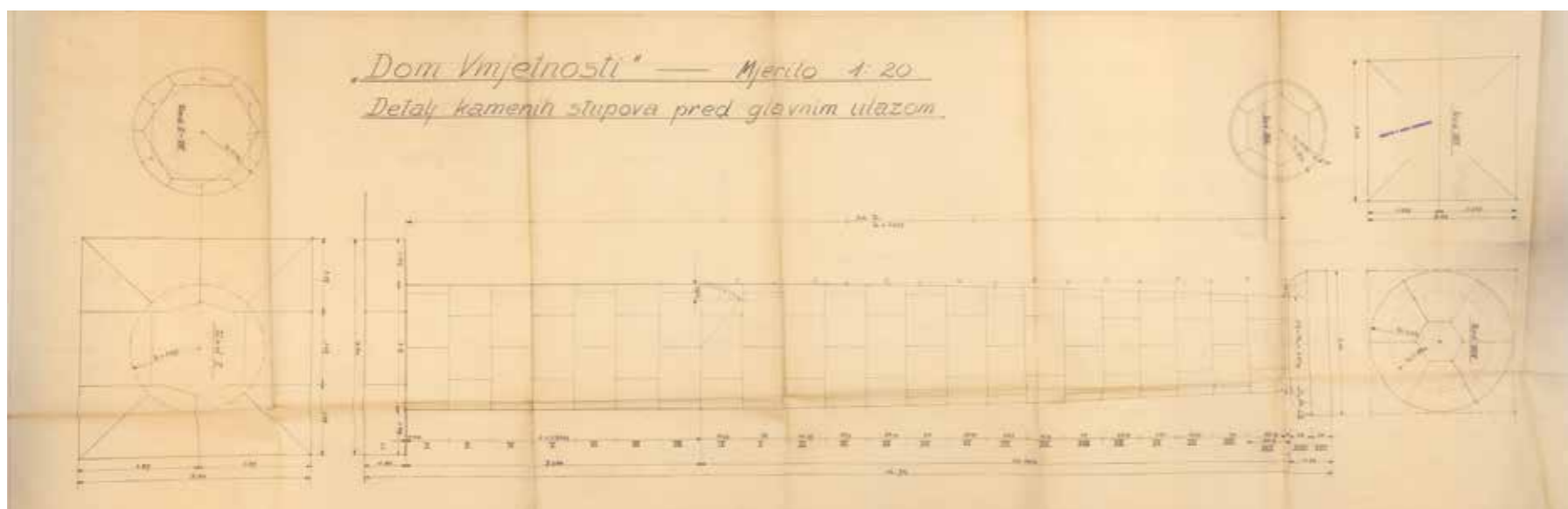
Nacrt detalja kamenih stupova pred glavnim ulazom, DAZG
